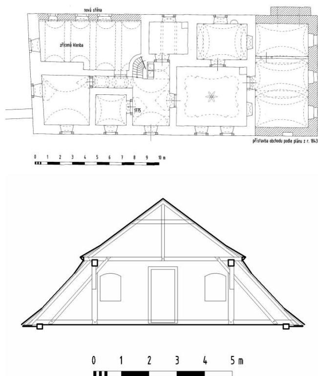
▲ Obr.15 : Půdorys současného přízemí a řez nepravým mansardovým krovem domu No.29 / dnes čp.19 (kresba autor 2018)
