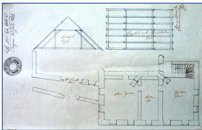
Obr. 21 : Plán úpravy domu No. 9 (zbořen po roce 1952) rozšířením o obytnou místnost v průčelí z roku 1837, před pozdější rekonstrukcí na hostinec (citace v pozn. 46).
