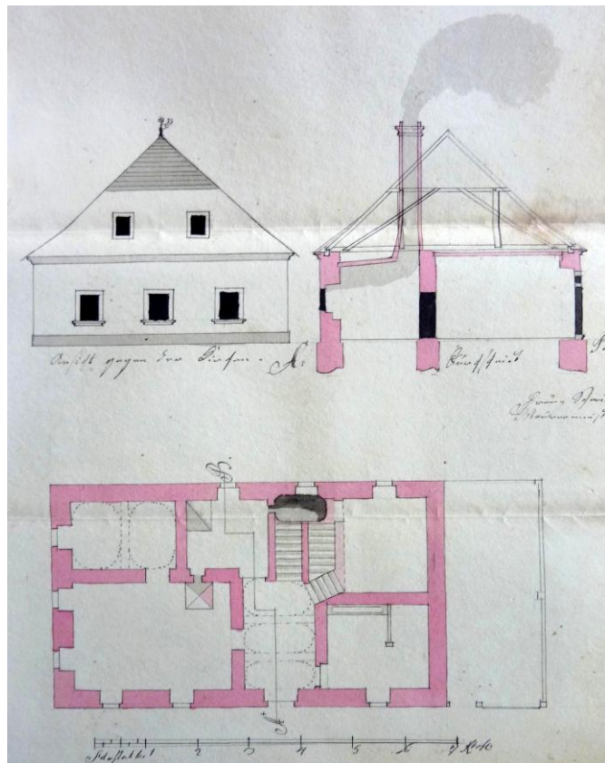
Obr. 34 : Plán na novostavbu domu No. 53 / dnes čp. 4 pro kameníka Josefa Poigera z roku 1842 (viz citace v pozn.65).
