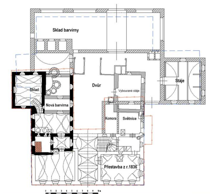
Obr. 25 : Plán přestavby domu No. 52 / dnes čp. 5 na patrovou budovu s okapovou orientací. Černé původní stav před rokem 1836 (patrně vybourán první díl od ulice s dřevěnými světnicemi), obrysy bez šraf – první přestavba z roku 1836, tečkované – vybourané stáje, šrafované objekty – další přestavba z roku 1842 (překresleno autorem z původních plánů do metrického měřítka) .
