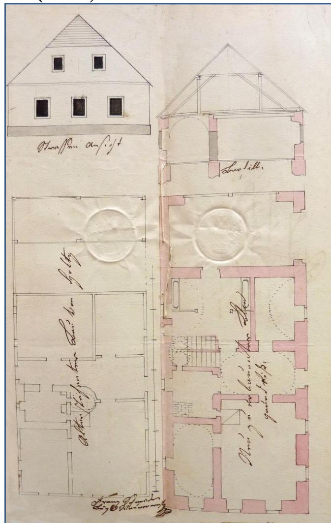
▲ Obr. 11 : Plán novostavby domu No. 47 (zbořen po roce 1952) z roku 1846 se zakreslením původního dřevěného domu s vyzděnou kuchyní a pecí (citace v pozn.23).
