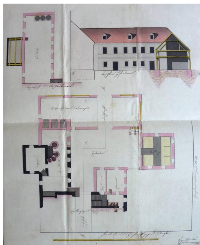
▲ Obr. 27 : Plán druhé přestavby domu No. 52 / dnes čp. 5 z r. 1842 s rozšířením barvířských provozů do patra zadního křídla a hospodářského zázemí (SOA Třeboň, odd. J. Hradec, fond Vs N. Bystřice, kart. 24, fol. 159).
