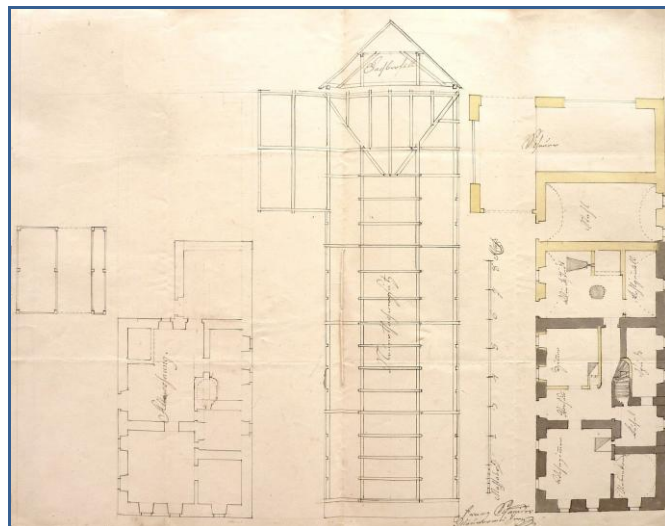
▲ Obr. 13 : Plán přestavby domu No. 41 s dalším doplněným číslem No. 86 z roku 1844 po předchozím požáru (nová část ještě žlutě) se zakreslením původního tvaru usedlosti (citace v pozn. 26).
