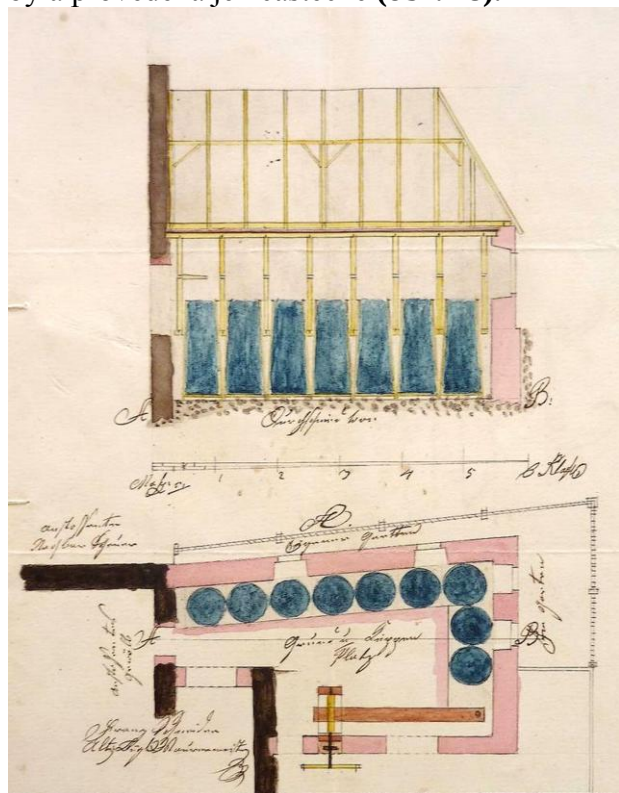
▲ Obr. 28 : Plán na přístavbu barviřské dílny z roku 1846 (citace v pozn. 56).
