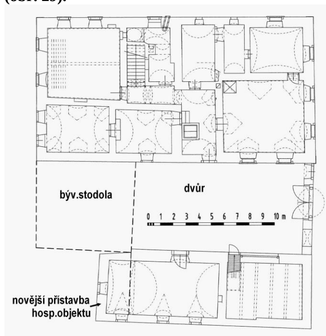
▲ Obr. 29 : Dispozice přízemí domu No. 33 / dnes čp. 18 po úpravách a nástavbě patra v roce 1839 (kresba autor)
