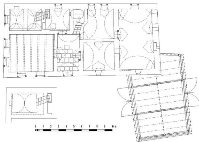
Obr. 35 : Dispozice přízemí domu se stodolou s No. 63 / dnes čp. 48 (kresba autor).
